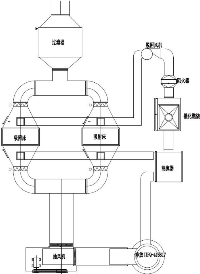
图 4.1-15 喷涂废气净化（含脱附）工艺示意图
