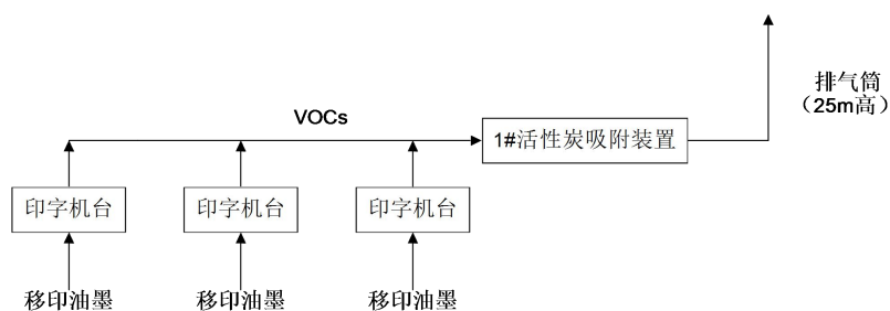
图 4.1-21 A 栋 4F 印字废气处理流程图
