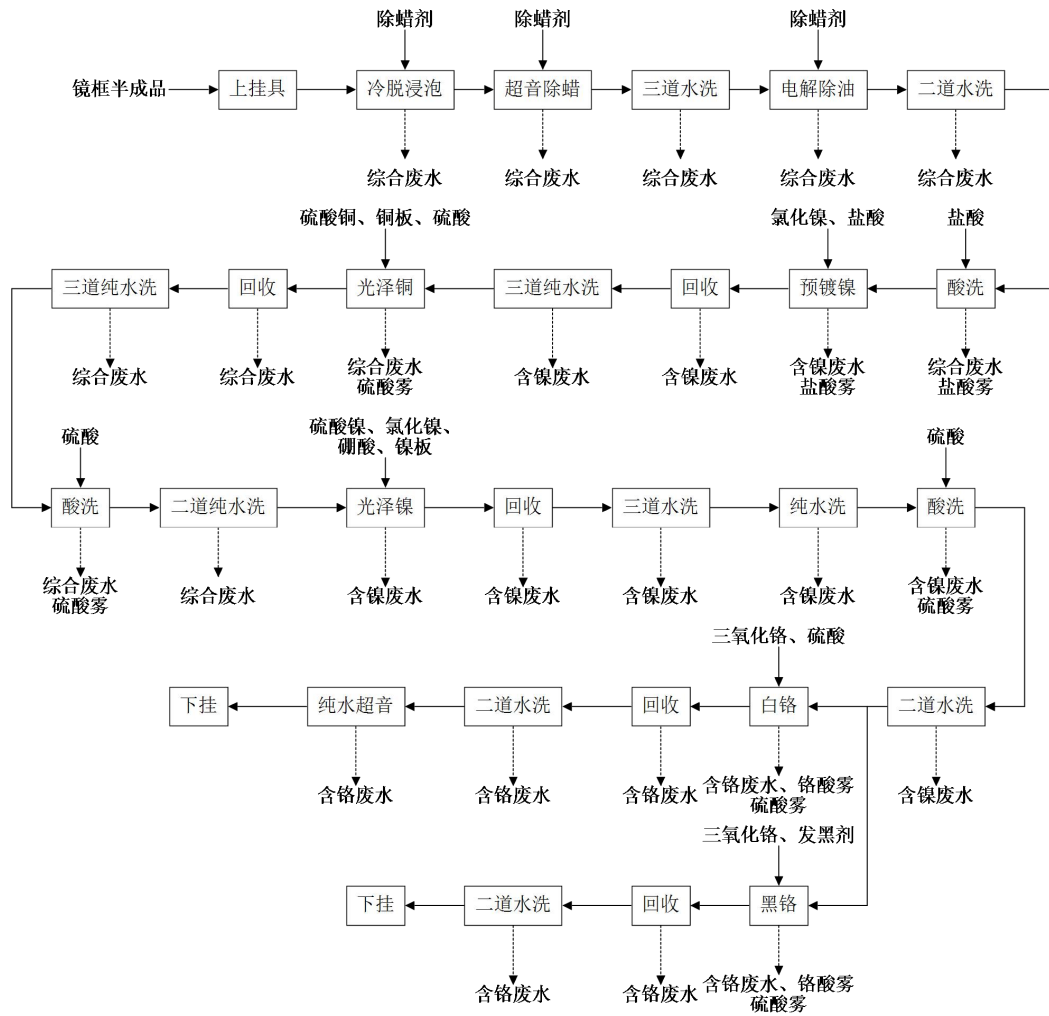
图 4.1-4 镀铬生产线工艺流程及产污环节示意图
