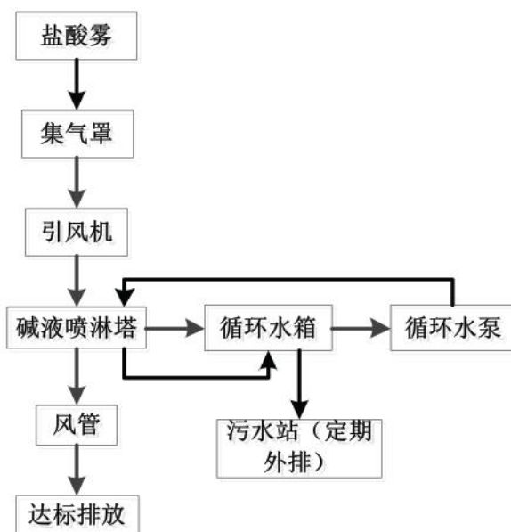
图 4.1-19 酸性废气塔工艺示意图
