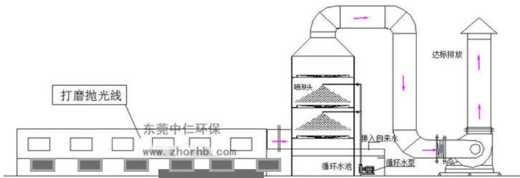
图 4.1-17 抛光粉尘处理工艺示意图
