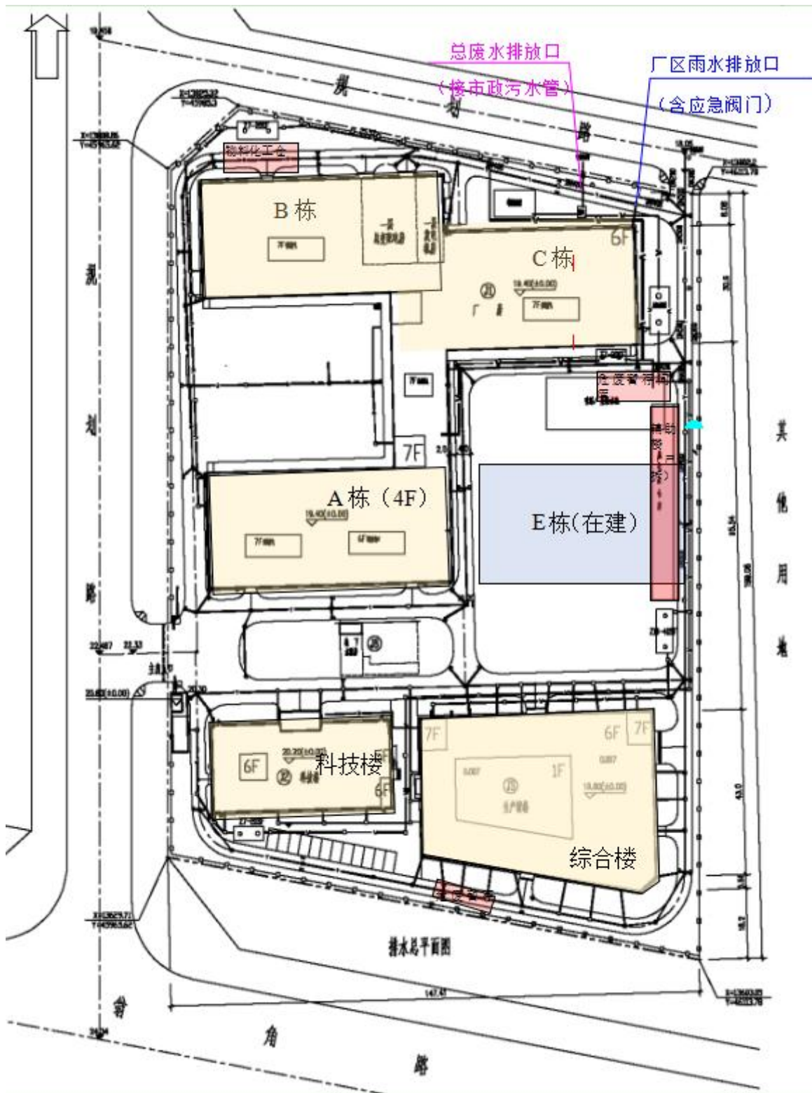
图 4.2-2 厂区雨污管网图
