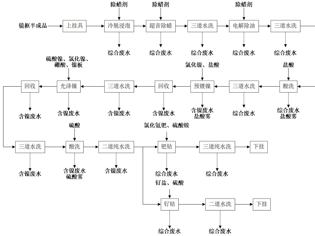
图 4.1-7 镀钯钉生产线工艺流程及产污环节示意图
